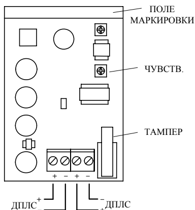
Рисунок 1 Схема подключения извещателя
