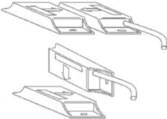
Рисунок 2. Варианты крепления датчиков
